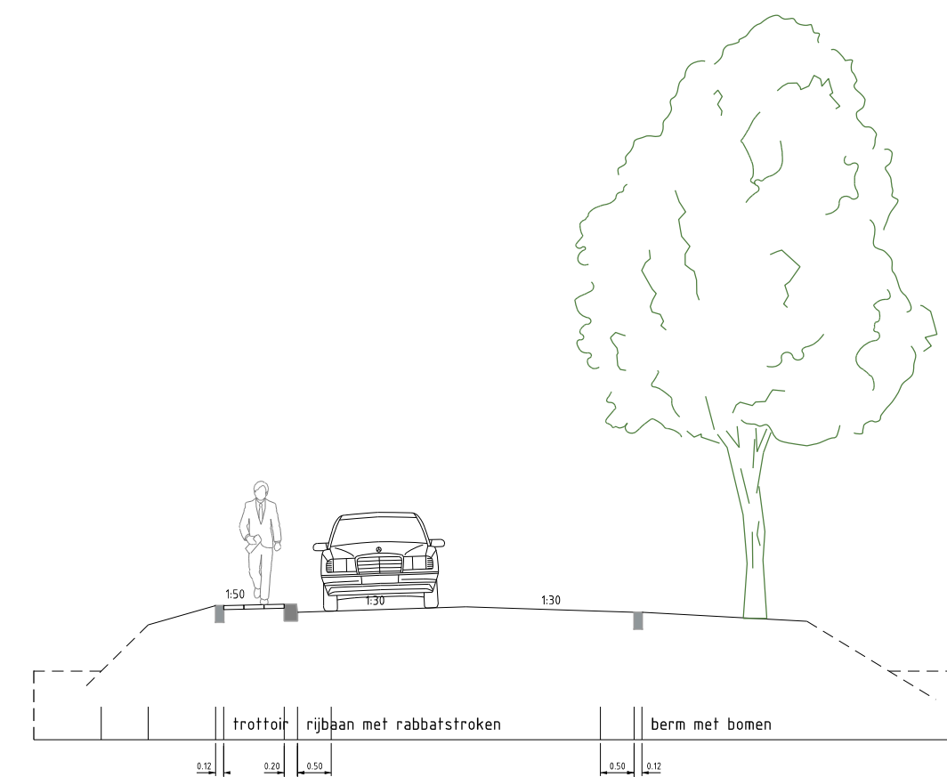
Principeprofiel B-B' (1:100)
