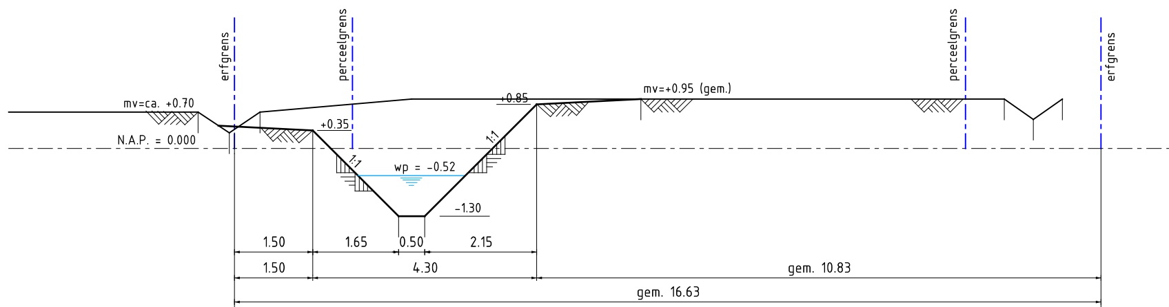
SITUATIE Schaal 1:500
