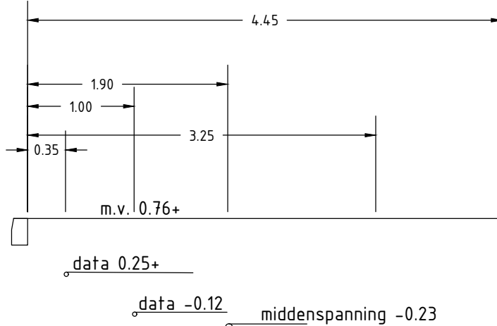
Doorsnede 2 proefsleuf kabels en leidingen schaal 1:50
