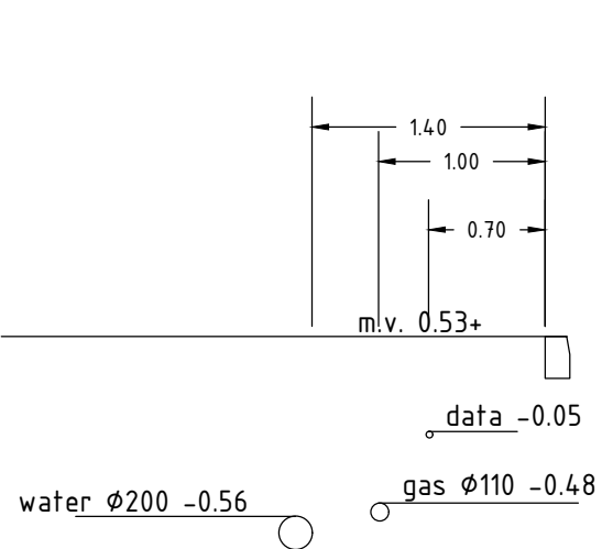
Doorsnede 1 proefsleuf kabels en leidingen schaal 1:50
