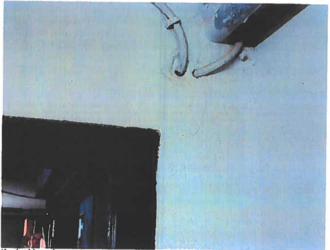
Voorbeeld van doorvoeringen die onvoldoende gedicht zijn met een brandwerend materiaal (behoort tot punt 1.2 en 1.3)
