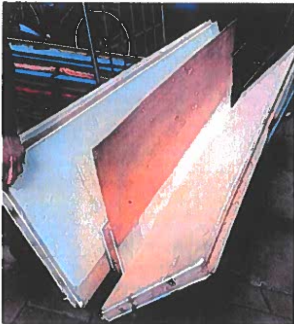
Het aanwezige restmateriaal van het merk Faay type VP54 waaruit de scheidingsconstructie is opgebouwd
