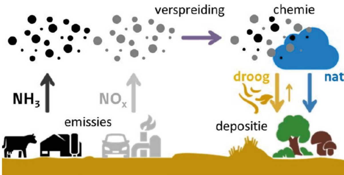
Figuur 10. Van emissie naar concentratie naar immissie/depositie
